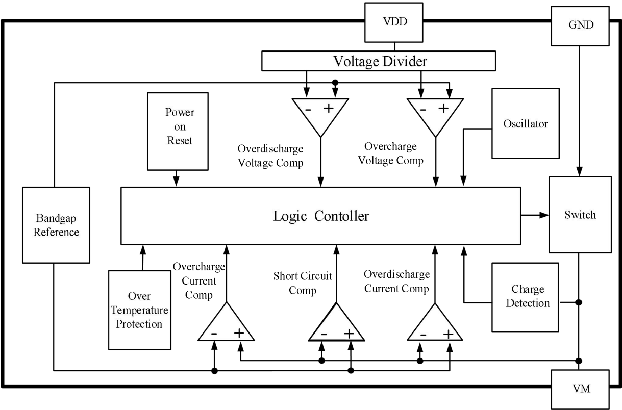
图 3 功能框图
