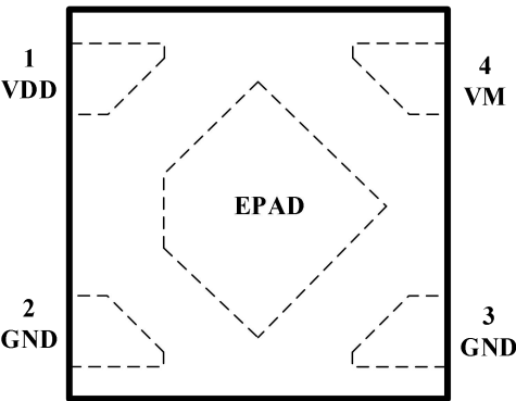
图 2 引脚定义
