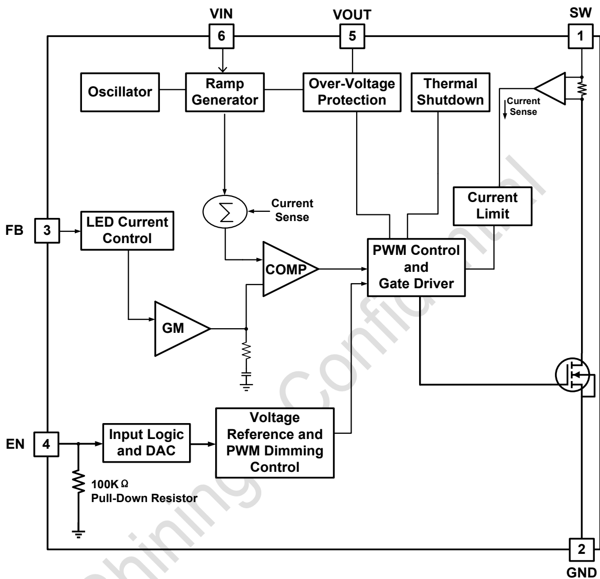
图 2.内部逻辑框图
