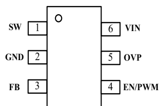
SOT23-6
