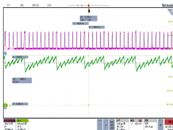
SW 最大限流(Ilimit) CH3:Vsw,CH4:Isw_max
