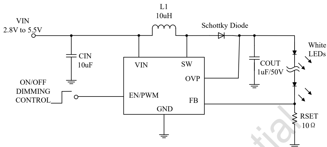
典型应用电路
